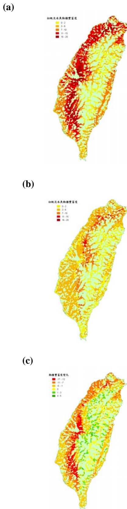
圖 5、以 GARP 導出的初級淡水魚物種豐富度預測：(a) 現今分布，(b) RSM2 情境下之分布，(c) 分布變化
